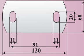
120x60 mm Malzeme 6 mm Ürün Kodu: 1141
