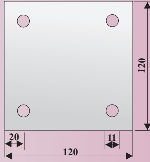
120x120 mm Malzeme 6 mm Ürün Kodu: 1144
