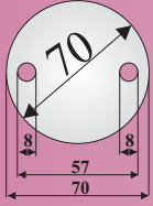
Ürün Kodu: 1120 Malzeme 4 mm
