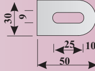
50x30 mm Malzeme 4 mm Ürün Kodu: 1151
