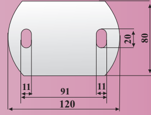
120x80 mm Malzeme 6 mm Ürün Kodu: 1142
