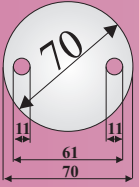
Ürün Kodu: 1121 Malzeme 6 mm, 11 mm Delikli
