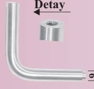
Montaj Kolu, ø 12 mm 75 x 75 mm M6 İç Dişli ve Kaynak için Ürün Kodu: 1226
