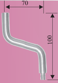
Montaj Kolu, ø 12 mm M8 Dış Dişli Ürün Kodu: 1229 M6 İç ve M8 Dış Dişli Ürün Kodu:1229-G
