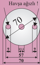
Ürün Kodu: 1130 Malzeme 4 mm, Orta Delik 12,1 mm , 9 mm Yan Delikler
