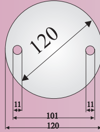
Ürün Kodu: 1124 Malzeme 6 mm, 11 mm Delikler
