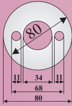
Ürün Kodu: 1131 Malzeme 6 mm, Orta Delik 34 mm ve 11 mm Yan Delikler
