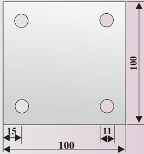
100x100 mm Malzeme 6 mm Ürün Kodu: 1143
