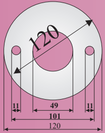
Ürün Kodu: 1133 Malzeme 6 mm, Orta Delik 49 mm ve 11 mm Yan Delikler
