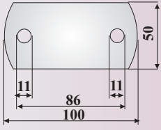
100x50 mm Malzeme 6 mm, 11 mm Delikler Ürün Kodu: 1140
