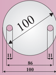
Ürün Kodu: 1123 Malzeme 6 mm
